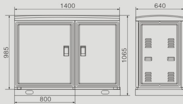
外形及安装尺寸图(mm)
